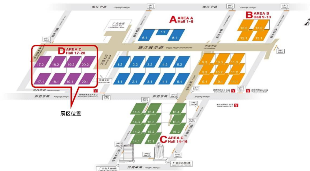
展区位置图
